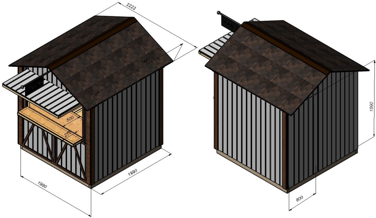
Эскизный план.
